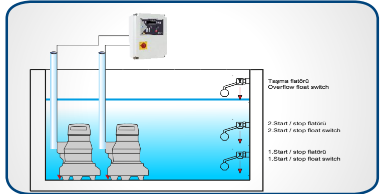
H-02/H-02M V2 İKİ POMPALI ATIK SU DALGIÇ H-02/H-02M V2 DUPLEX SUBMERSIBLE PUMP
